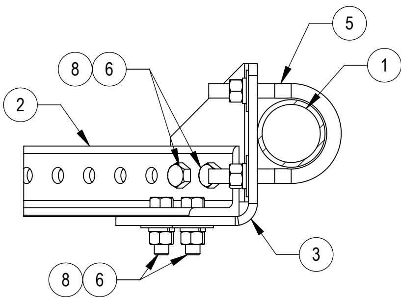
SECTION B-B SCALE 1 : 4
