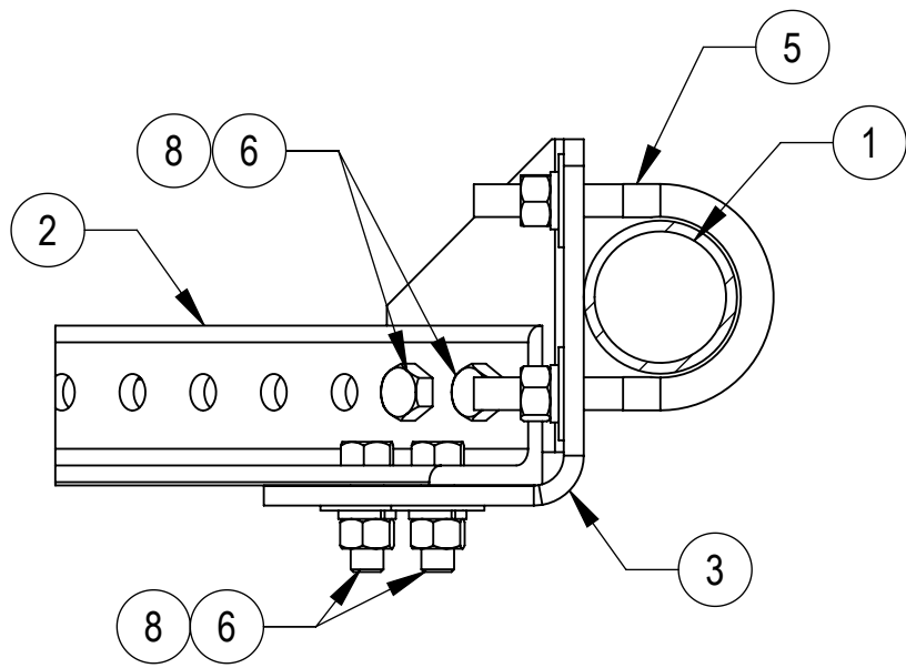
SECTION B-B SCALE 1 : 4
